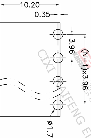
P.C.B.LAYOUT
