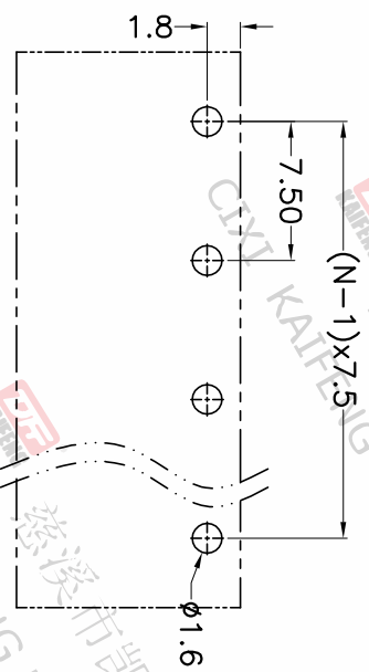
P.C.B.LAYOUT
